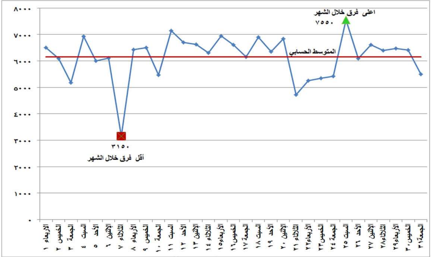
شكل (٣) الفرق بين أقصى وأدنى حمل خلال شهر أغسطس ٢٠١٨
