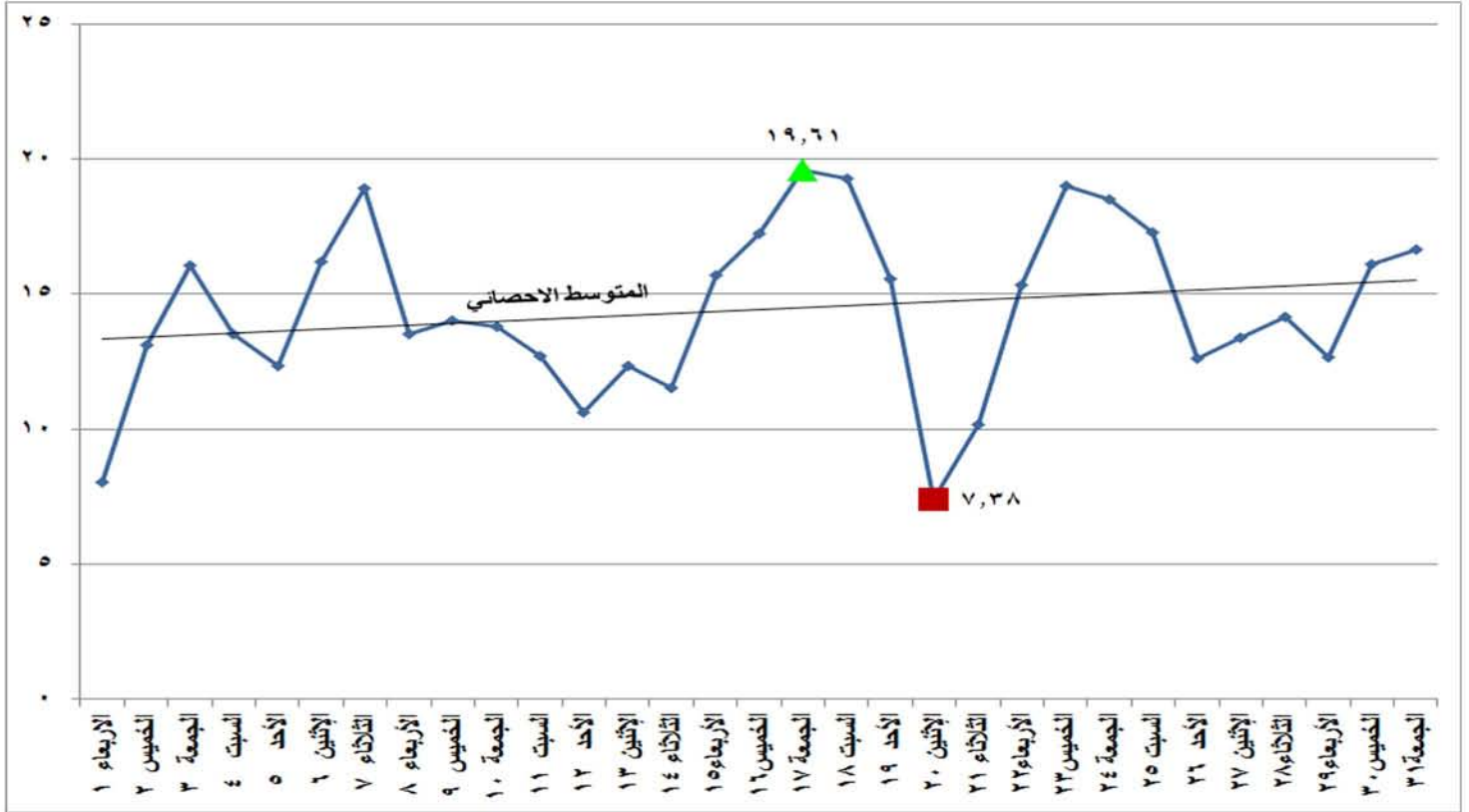
شكل (٢٥) الطاقة الكهربائية المنتجة من الرياح والشمس خلال شهر أغسطس ٢٠١٨
