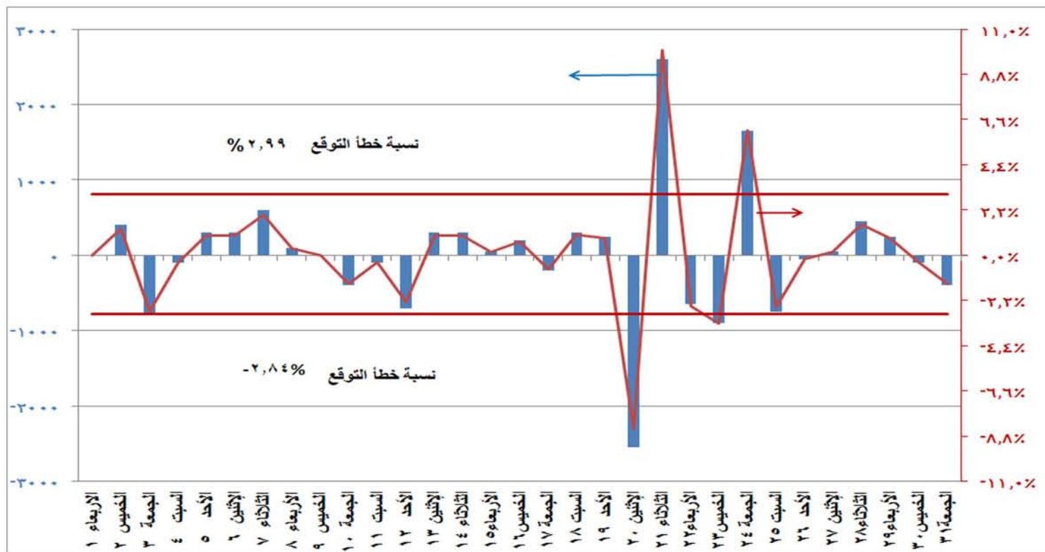
شكل (١٠) الفرق بين الحمل الأقصى المتوقع والمسجل فعليا ونسبة الفرق الى الحمل المسجل فعليا خلال شهر أغسطس ٢٠١٨
