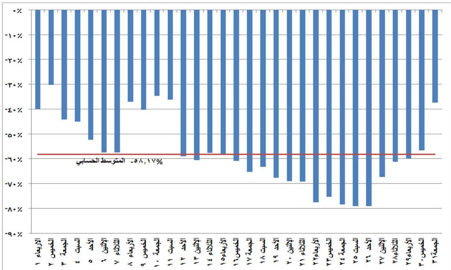
شكل (٢٠) نسب التغير في استخدام المازوت في إنتاج الطاقة الكهربائية خلال شهر أغسطس ٢٠١٨ مقارنة بالشهر المماثل من العام السابق
