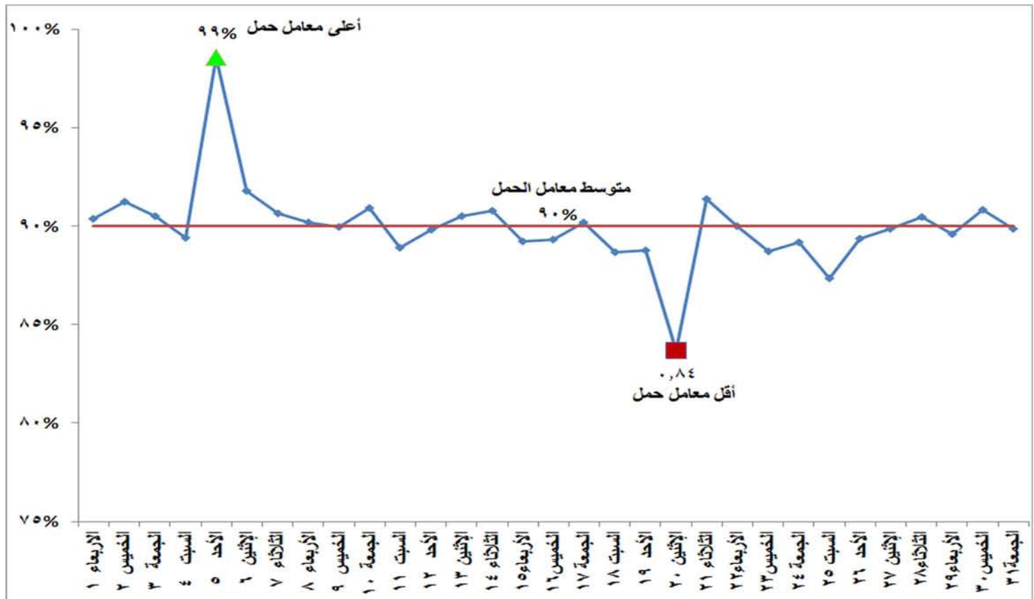
شكل (١٢) إجمالي معامل الحمل لوحدات الانتاج خلال شهر أغسطس ٢٠١٨
