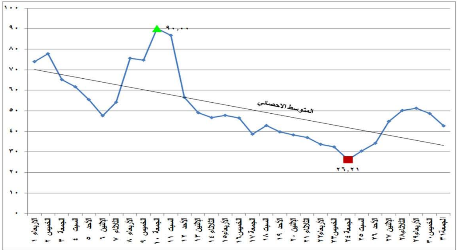
شكل (١٩) الطاقة الكهربائية المنتجة من المازوت خلال شهر أغسطس ٢٠١٨
