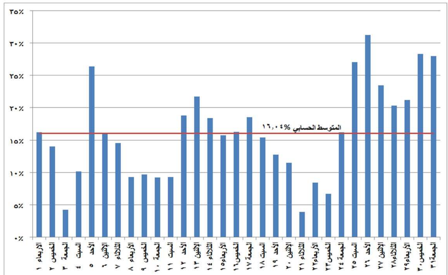
شكل (١٨) نسب التغير في استخدام الغاز الطبيعي في إنتاج الطاقة الكهربائية خلال شهر أغسطس ٢٠١٨ مقارنة بالشهر المماثل من العام السابق
