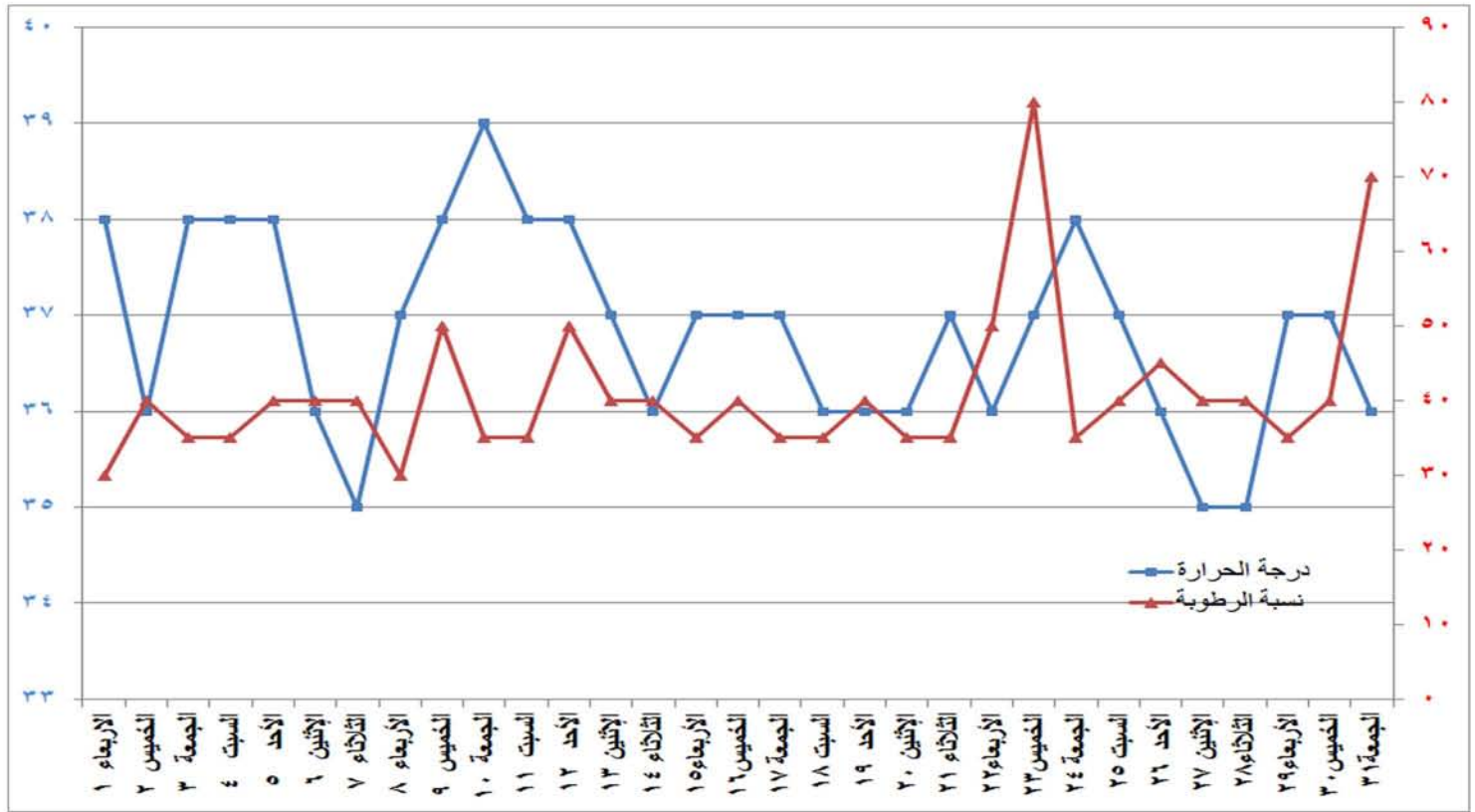
شكل (١١) التغيير في درجة الحرارة والرطوبة النسبية خلال شهر أغسطس ٢٠١٨
