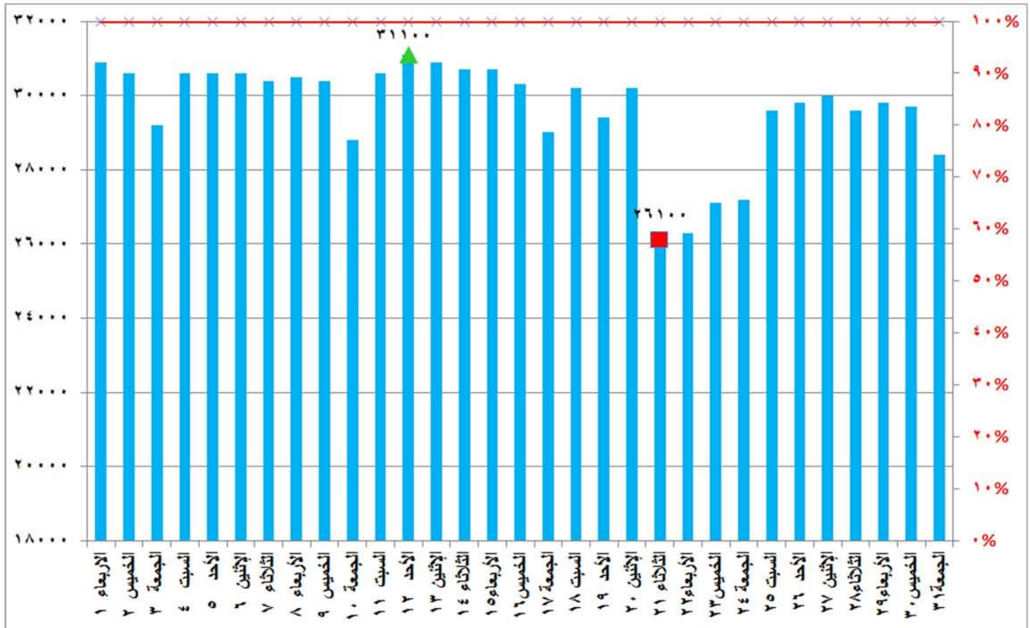
شكل (٥) قدرات الانتاج المتاحة ونسبتها للحمل الأقصى خلال شهر أغسطس ٢٠١٨
