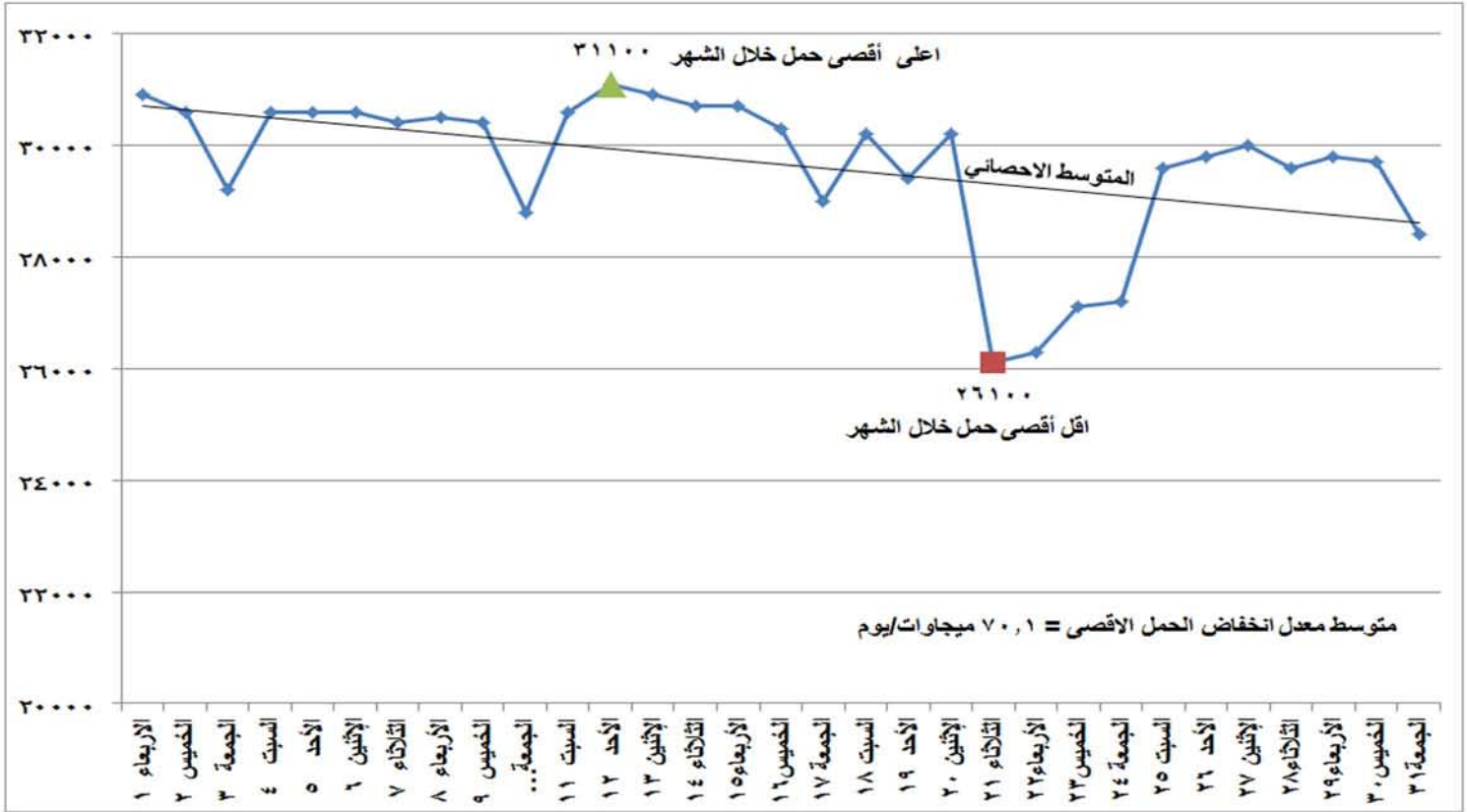
شكل (١) تطور الحمل الاقصى اليومي خلال شهر أغسطس ٢٠١٨
