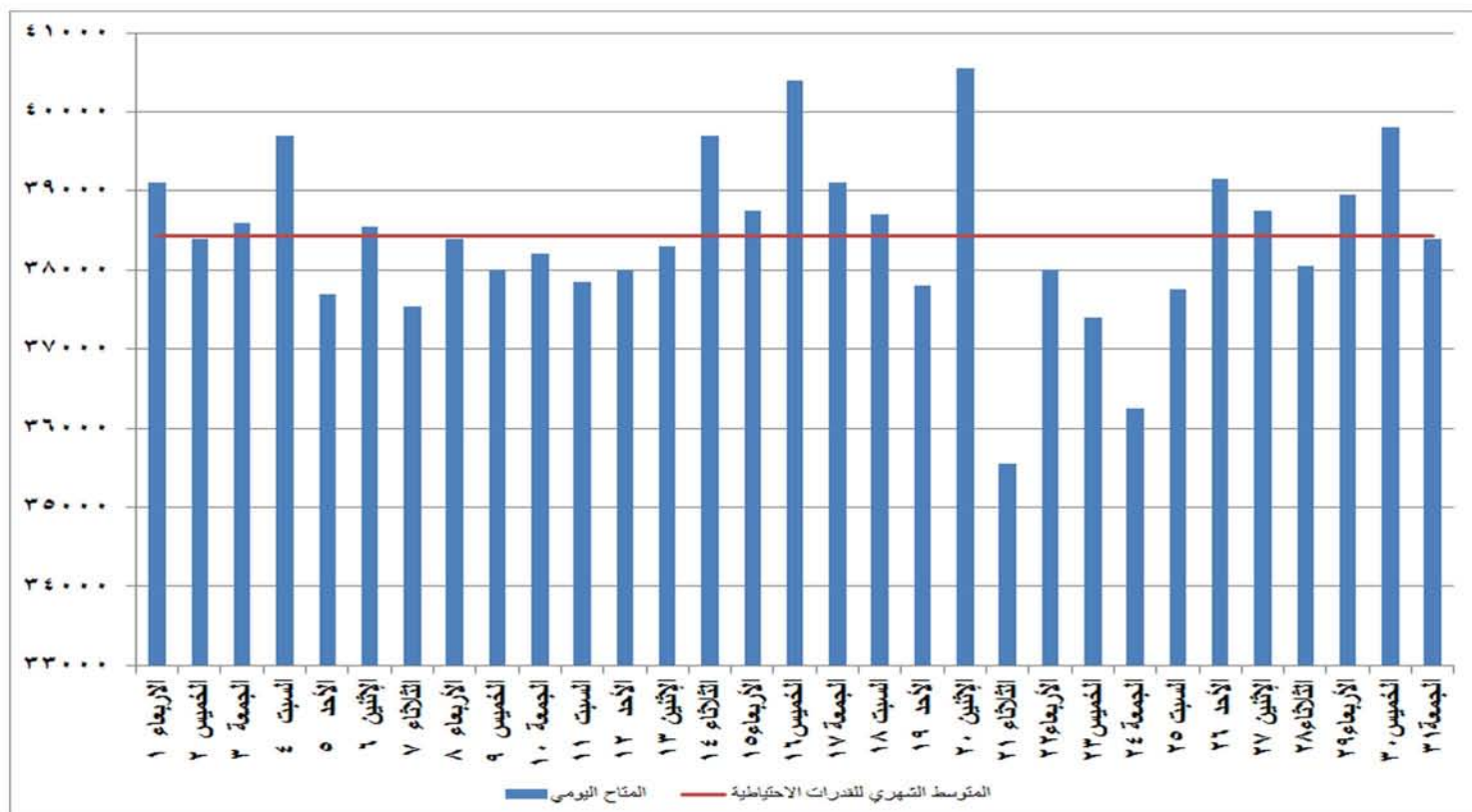
شكل (٢٧) القدرات المتاحة يوميا والمتوسط الشهري للقدرة الاحتياطية خلال شهر أغسطس ٢٠١٨
