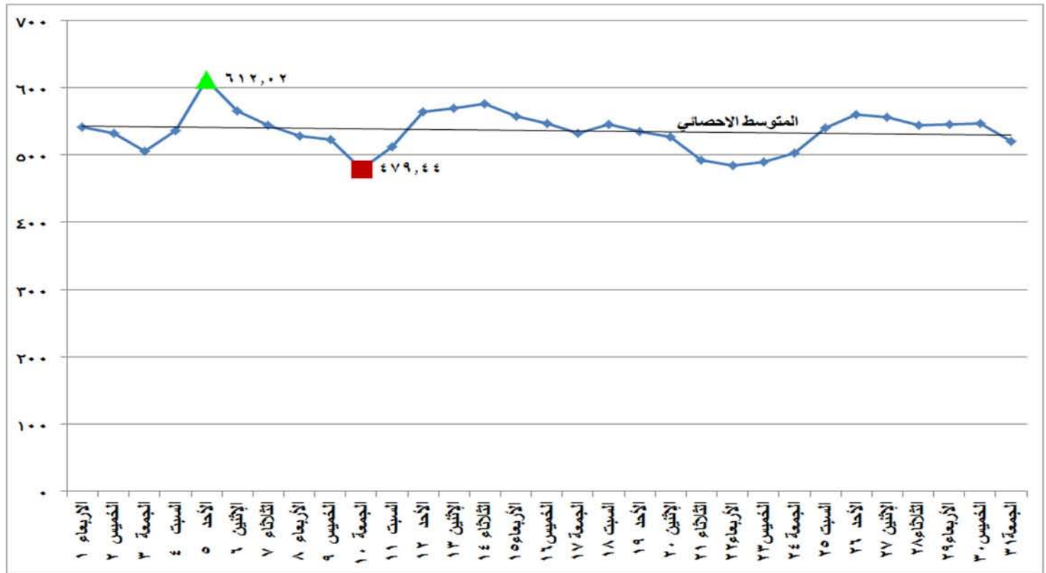
شكل (١٧) الطاقة الكهربائية المنتجة من الغاز الطبيعي خلال شهر أغسطس ٢٠١٨
