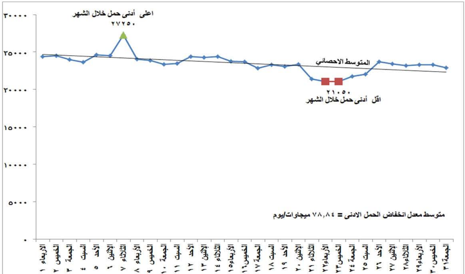
شكل (٢) تطور الحمل الادنى اليومي خلال شهر اغسطس ٢٠١٨
