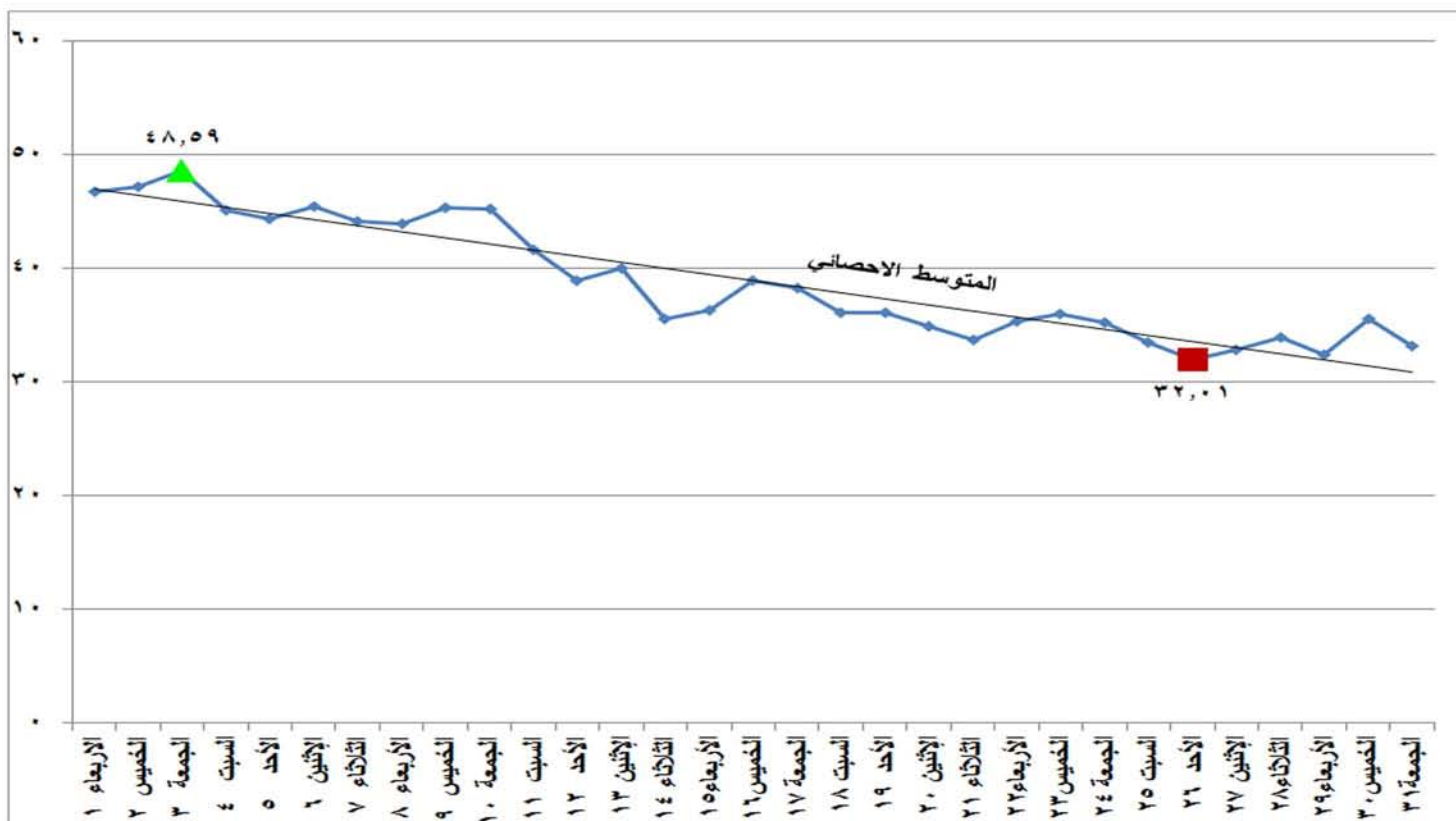
شكل (٢٣) الطاقة الكهربائية المنتجة من المصادر المائية خلال شهر أغسطس ٢٠١٨
